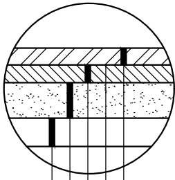
7 TON BITUMINOUS PATCH (<1000 ADT) SANDY SOILS (AASHTO SOILS A-1, A-2)
