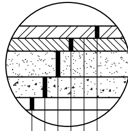
7 TON BITUMINOUS PATCH (<1000 ADT) CLAY SOILS (AASHTO SOILS A-6, A-7)
