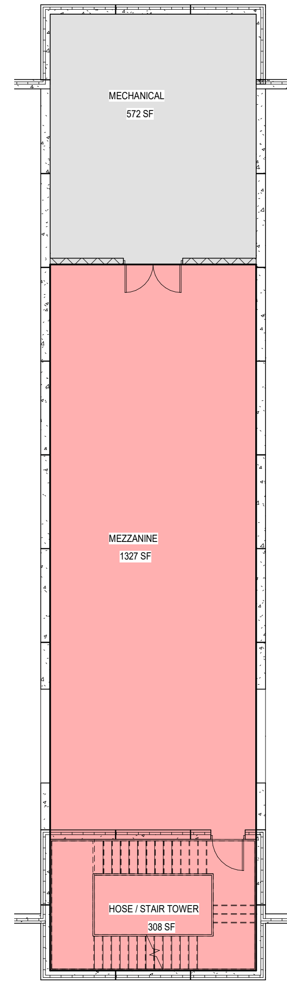
2 MEZZANINE PLAN SCALE: 1" = 10'-0"
